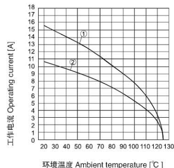
① 24B 外壳 带 6 个模块, 导线截面 Wire gauge: 2.5 mm 2 ② 24B 外壳 带 6 个模块, 导线截面 Wire gauge: 1.5 mm 2
