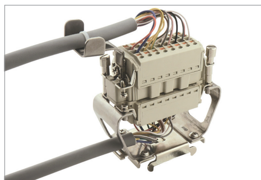
6: 安装绑线架
