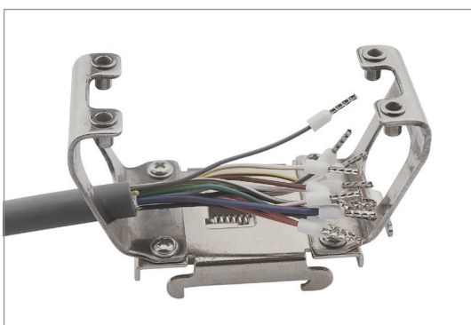
2: 穿线
