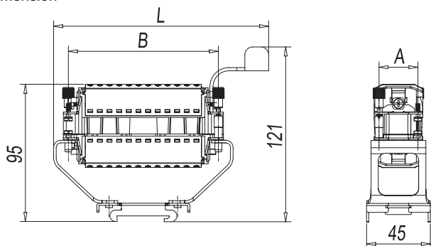
尺寸图 Dimension
