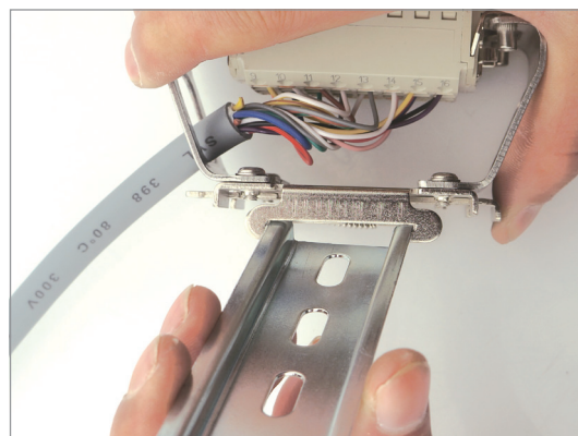
7: 卡入导轨
