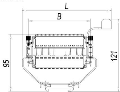
尺寸图 Dimension
