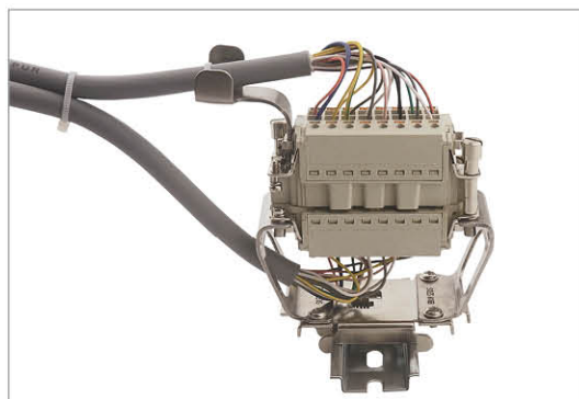
8: 完成安装
