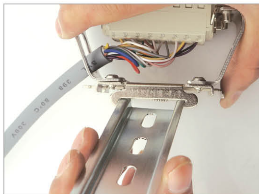
7: 卡入导轨
