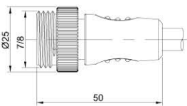
插针 Male 直出 Straight
