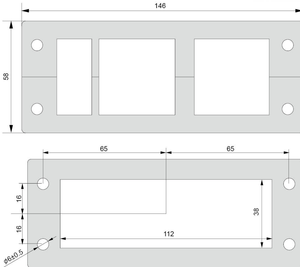
开孔尺寸 Size
