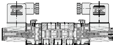
双电控电磁阀
