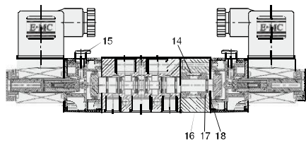
三位置电磁阀
