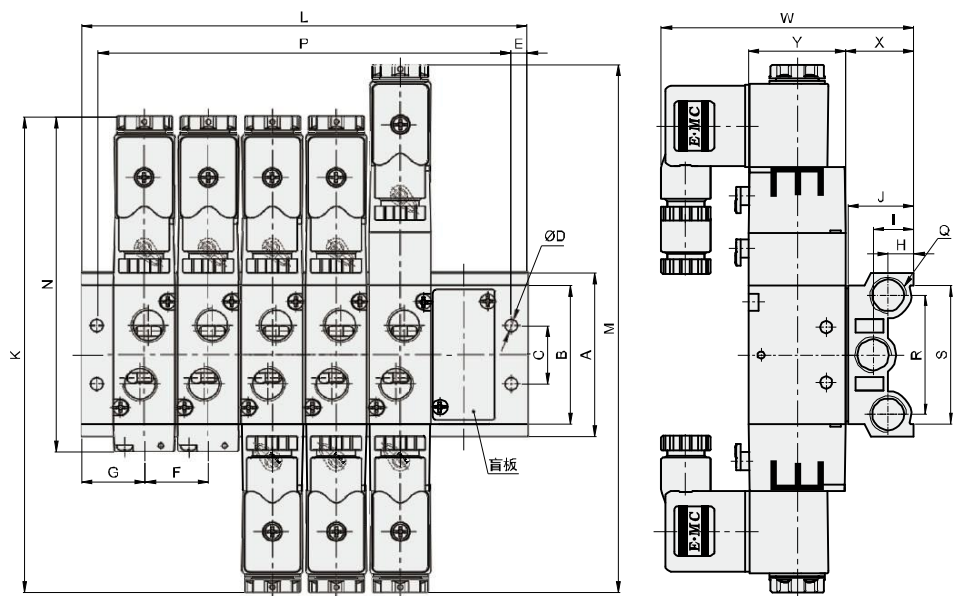
外形尺寸图
