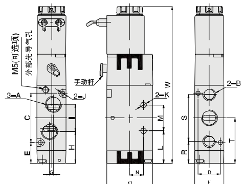
引出线式
