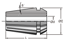
寸法 Dimension(mm)
