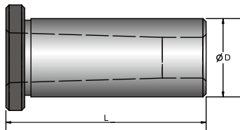
寸法 Dimension(mm)
