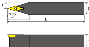
寸法 Dimension(mm)
