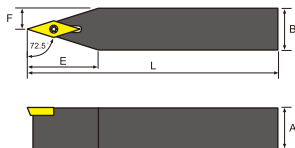
寸法 Dimension(mm)
