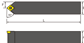
寸法 Dimension(mm)
